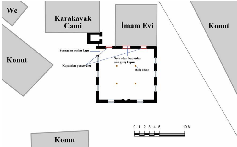
Şekil 11: Tarihi Karakavak Camii'nin planı ve konumu
