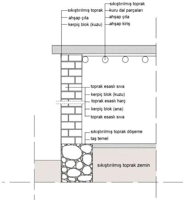
Şekil 5: Tek katlı kerpiç bir yapının strüktürel kesit krokisi
