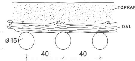
Şekil 6: Kerpiç yapı üst örtü sistemi detayı
