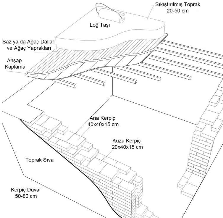
Şekil 12: Yığma sistem düz damlı kerpiç bir yapının aksometrik görünüşü
