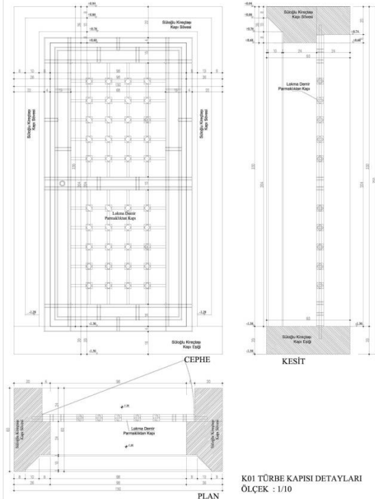
Şekil 17. Kâbü'lî Mustafa Efendi Türbesi Niyaz Penceresi ile Türbe Harim Kısmı Kapısı Detay
