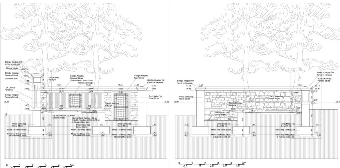
Şekil 11. Kâbüli Mustafa Efendi Türbesi Koruma Projesi, B-B / C-C Kesitleri
