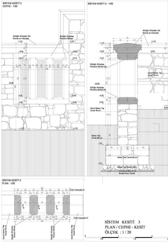
Şekil 15. Kâbü'lî Mustafa Efendi Türbesi Koruma Projesi, Moloz Taş Duvar – Pencere Detay
