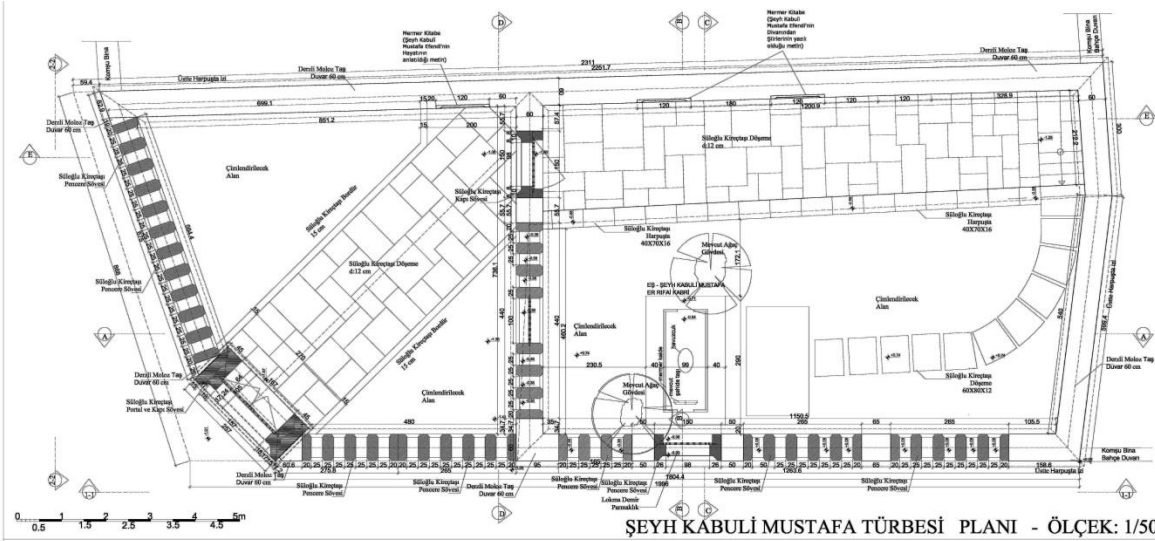
Şekil 9. Kâbüli Mustafa Efendi Türbesi Koruma Projesi, Plan
