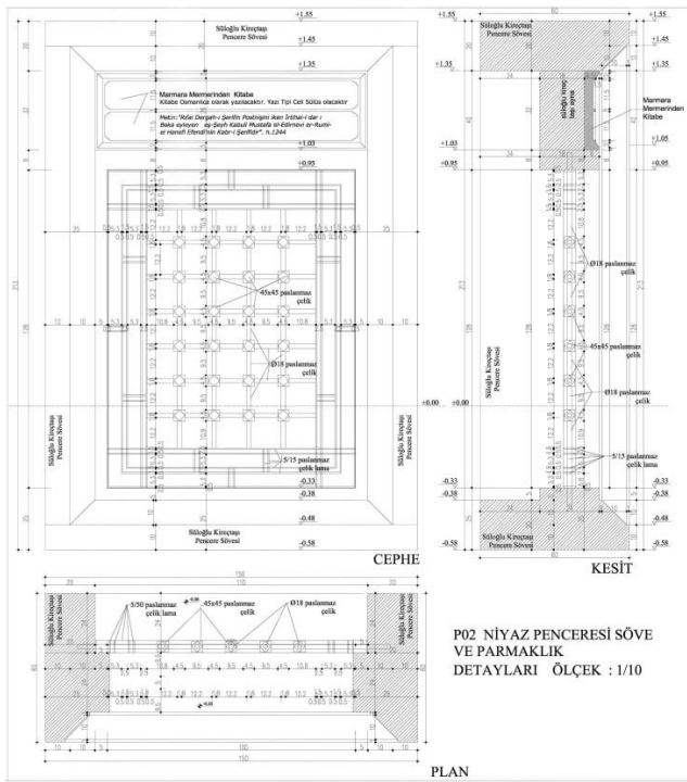
Şekil 17. Kâbü'lî Mustafa Efendi Türbesi Niyaz Penceresi ile Türbe Harim Kısmı Kapısı Detay
