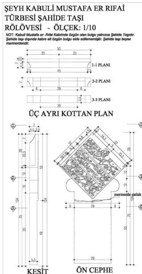
Şahide Taşı Rölövesi
