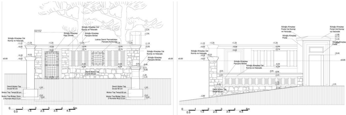
ŞEYH KABULİ MUSTAFA TÜRBESİ D-D KESİTİ - ÖLÇEK: 1/50
