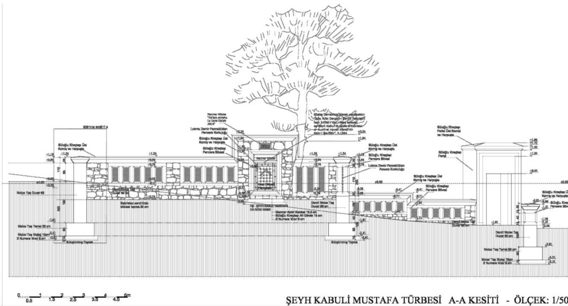
Şekil 10. Kâbüli Mustafa Efendi Türbesi Koruma Projesi, A-A Kesiti
