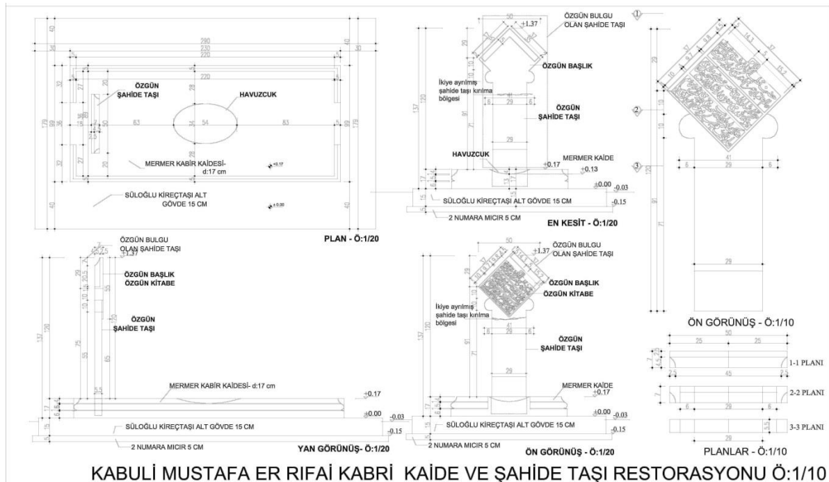
Şekil 14. Kâbüî Mustafa Efendi Türbesi Kabir Kaidesi ve Şahide Taşı Restorasyonu Projesi
