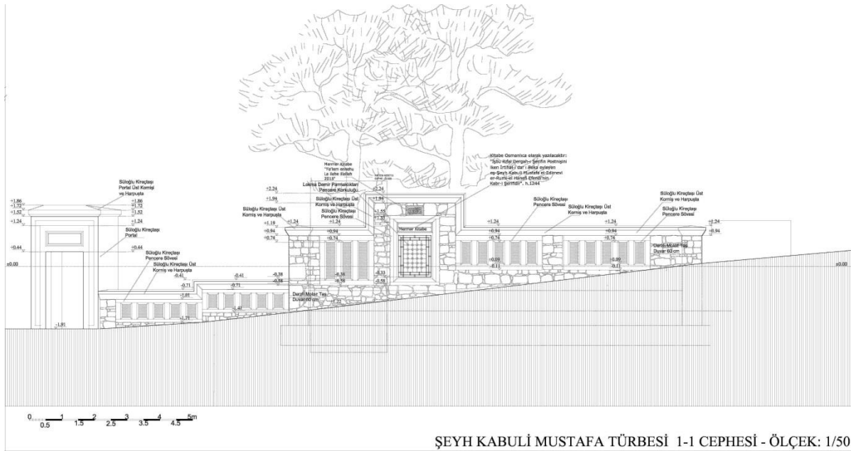
Şekil 12. Kâbüî Mustafa Efendi Türbesi Koruma Projesi, 1-1 Cephesi
