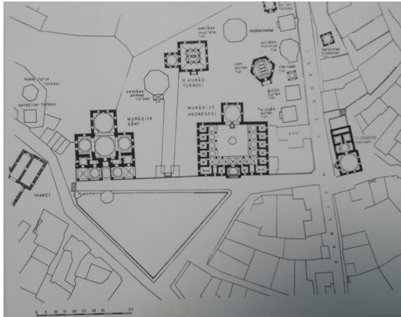
Şekil 8. Bursa, Muradiye Külliyesi Yerleşim Düzeni (Ayverdi 1989b)
