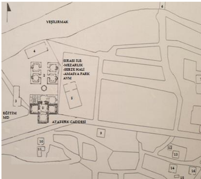
Şekil 1. Amasya Yörgüç Paşa Külliyesi, Restitüsyon Krokisi (Ölçeksiz) (Toruk 2002 üzerinden yeniden çizilerek güncellenmiştir)
