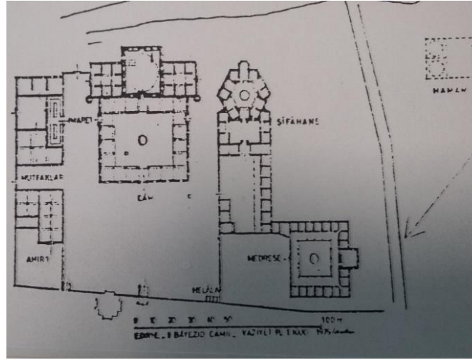
Şekil 10. Edirne II. Bayezid Külliyesi Yerleşim Düzeni (Yüksel 1983)
