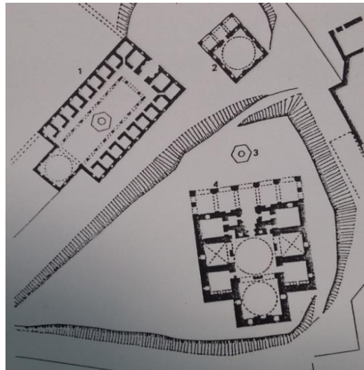
Şekil 6. Bursa Yıldırım Bayezid Külliyesi Yerleşim Düzeni (Goodwin 1993)
