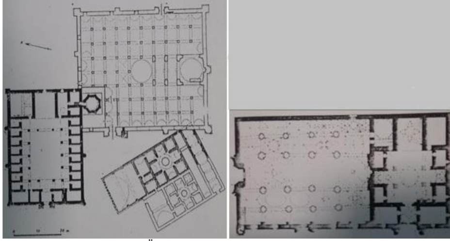
Şekil 4. Anadolu’da Erken Dönem Külliye Örnekleri A. Kayseri Huand Hatun Külliyesi Plan (Karamağaralı 1976), B. Divriği, Ulu Cami Külliyesi (A. Gabriel 1934)
