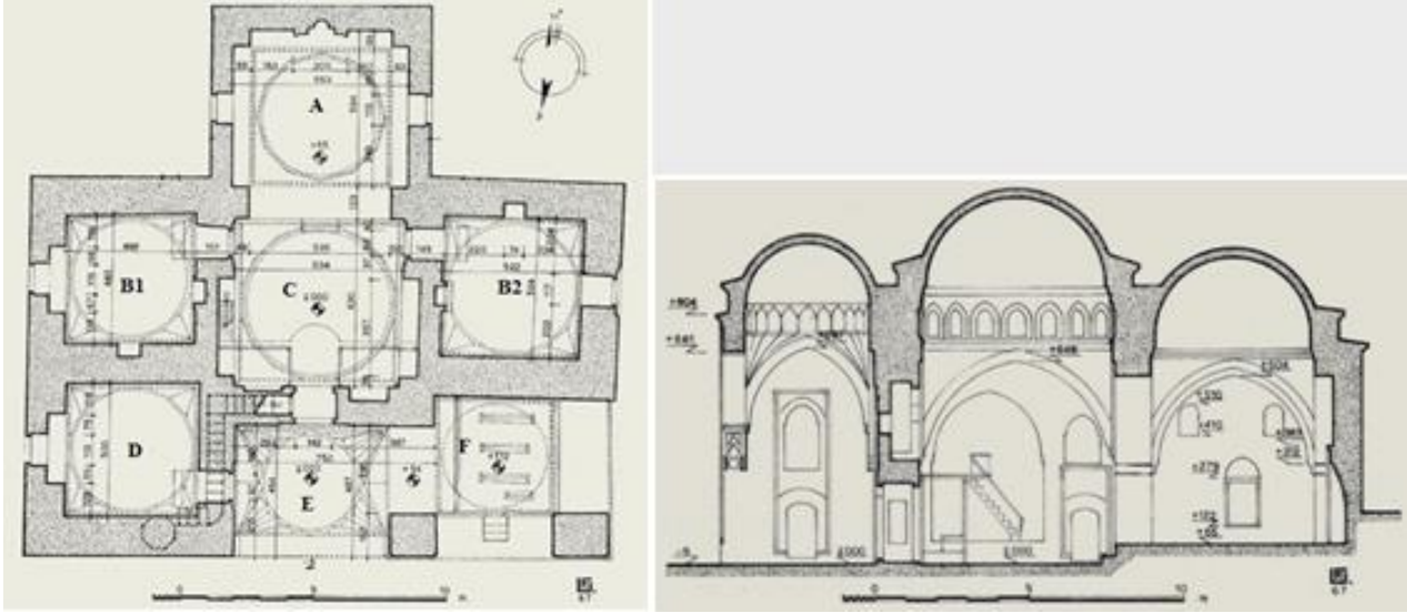
Şekil 2. Amasya Yörgüç Paşa Külliyesi Plan ve Kesit (Ayverdi 1989a)
